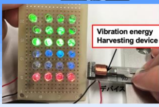
振動発電デバイス
